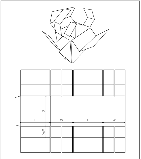
FEFCO 0208
