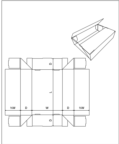
FEFCO 0437
