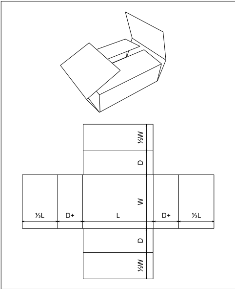
FEFCO 0402
