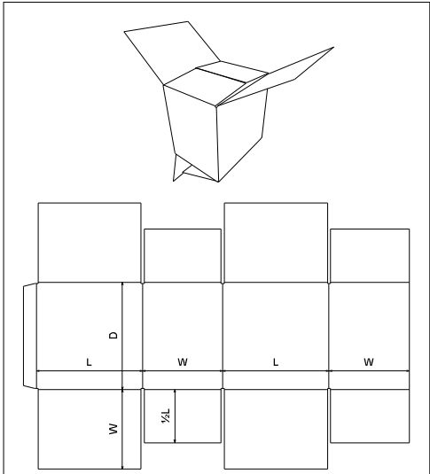
FEFCO 0206
