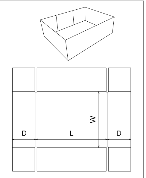
FEFCO 0911
