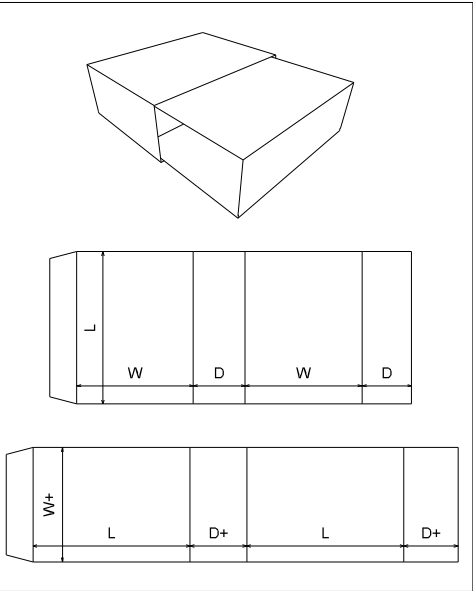
FEFCO 0505
