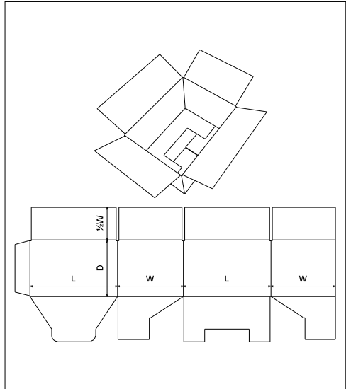
FEFCO 0216
