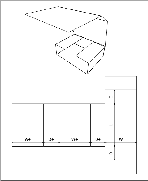
FEFCO 0400
