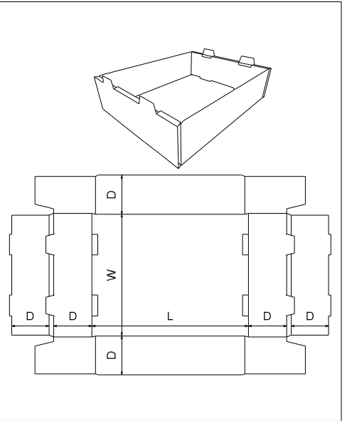
FEFCO 0435
