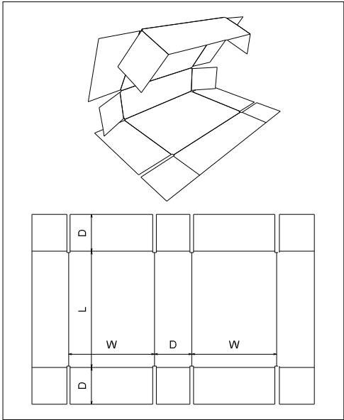
FEFCO 0409
