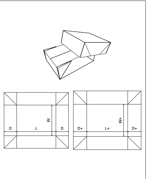
FEFCO 0309
