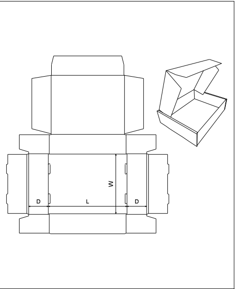
FEFCO 0429
