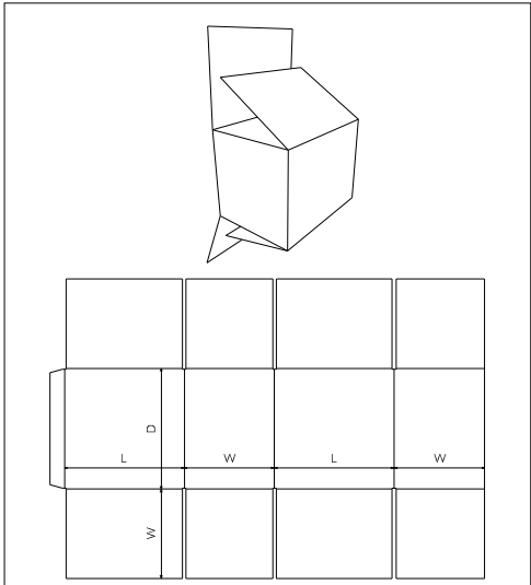
FEFCO 0203
