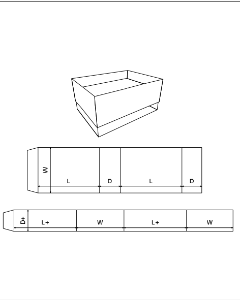
FEFCO 0504
