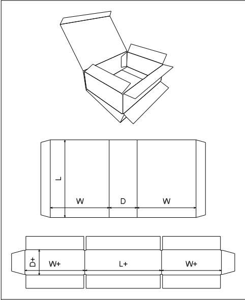
FEFCO 0512
