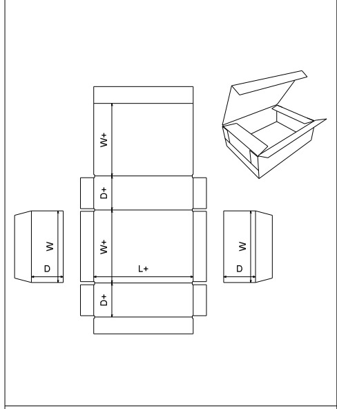
FEFCO 0602
