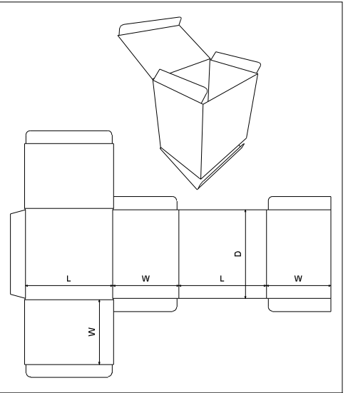
FEFCO 0210
