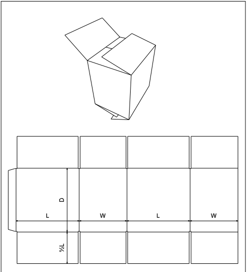
FEFCO 0205
