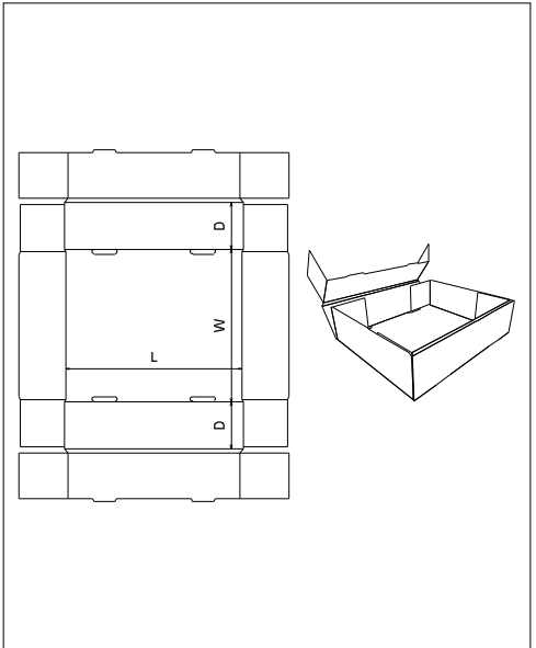
FEFCO 0424
