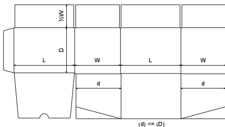
FEFCO 0225
