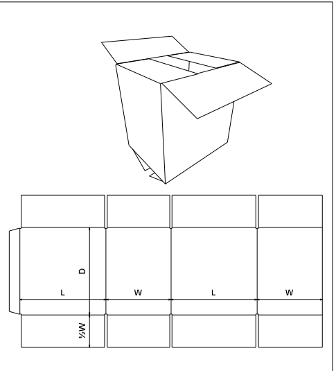
FEFCO 0201
