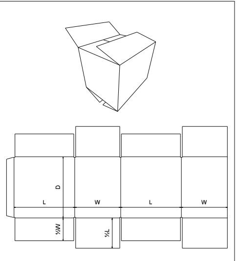
FEFCO 0204
