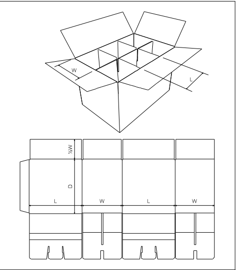
FEFCO 0207
