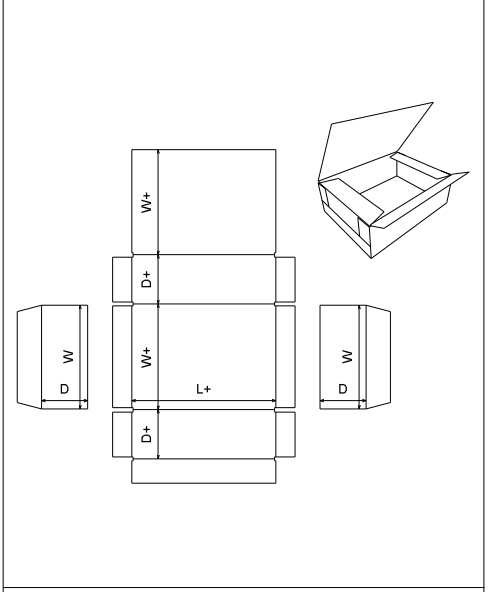
FEFCO 0601
