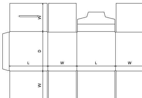
FEFCO 0218
