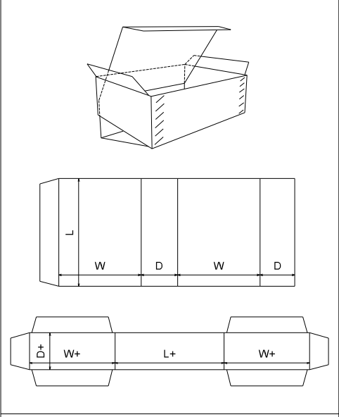
FEFCO 0511
