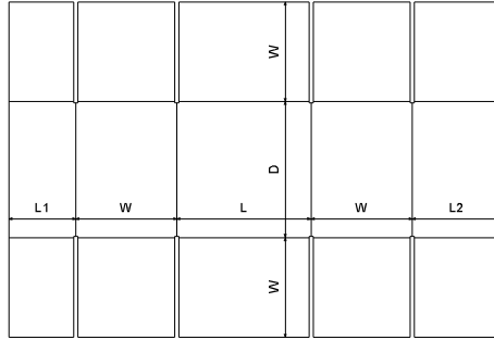
FEFCO 0230
