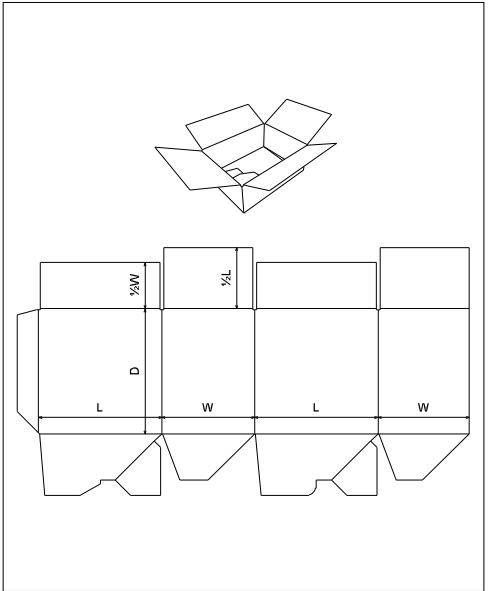
FEFCO 0712
