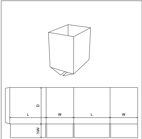
FEFCO 0200
