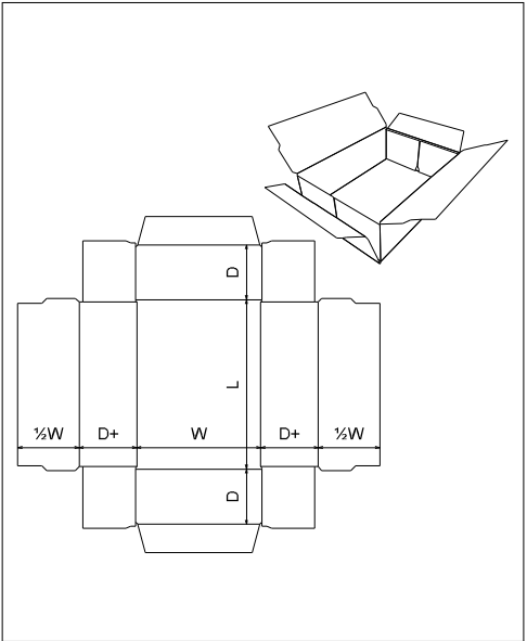
FEFCO 0415
