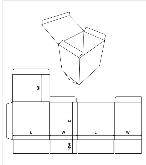
FEFCO 0212
