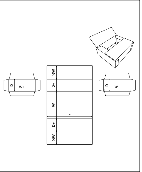
FEFCO 0605
