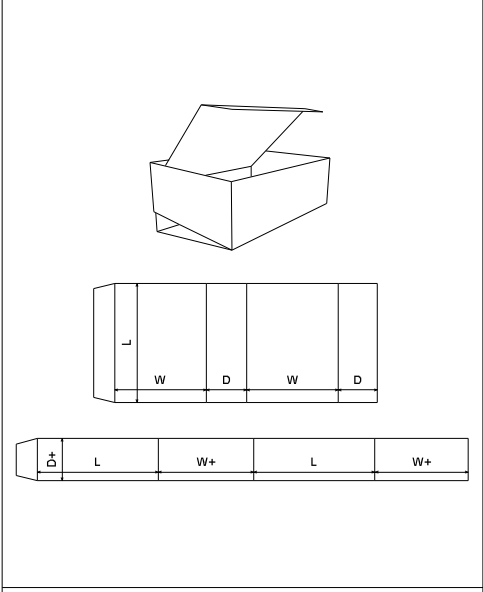
FEFCO 0510
