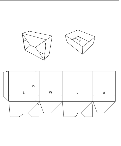
FEFCO 0700
