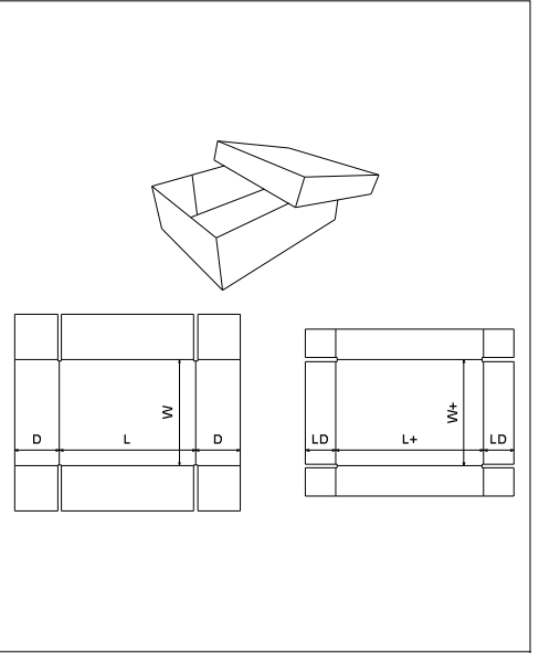
FEFCO 0306
