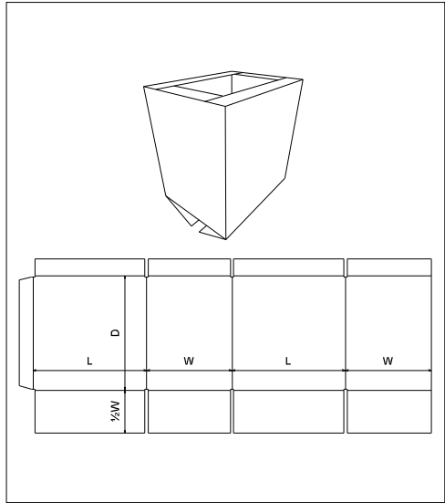
FEFCO 0209
