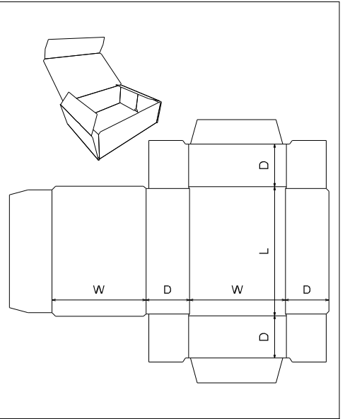
FEFCO 0420
