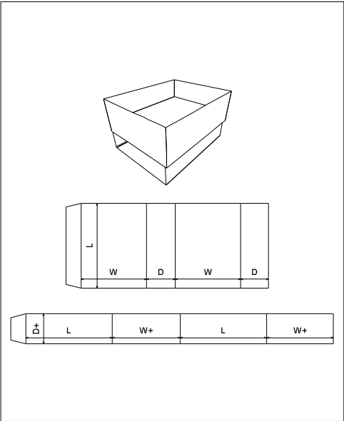
FEFCO 0507
