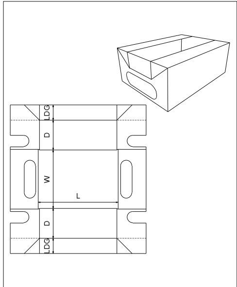
FEFCO 0434
