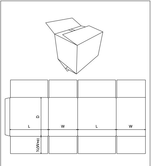
FEFCO 0202
