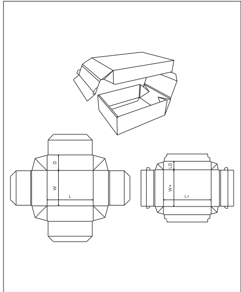
FEFCO 0323
