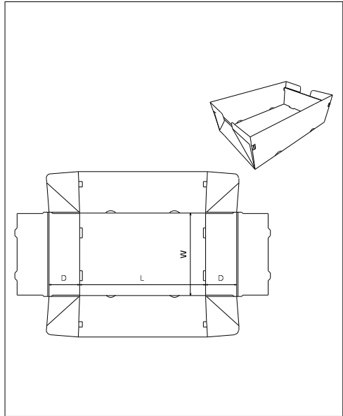
FEFCO 0772
