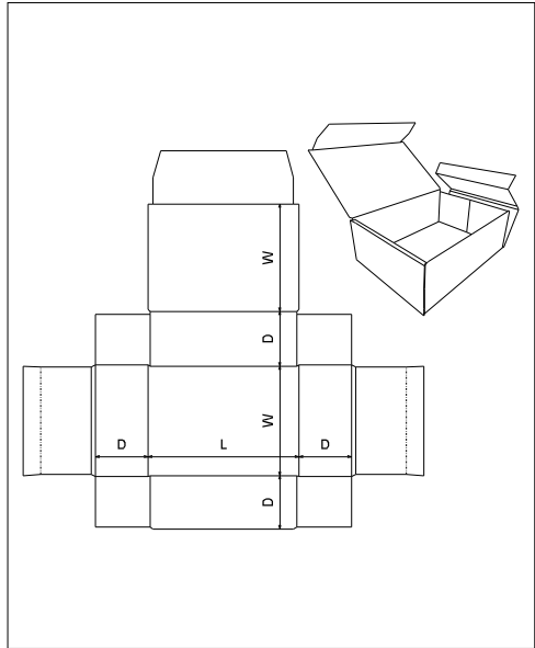
FEFCO 0428
