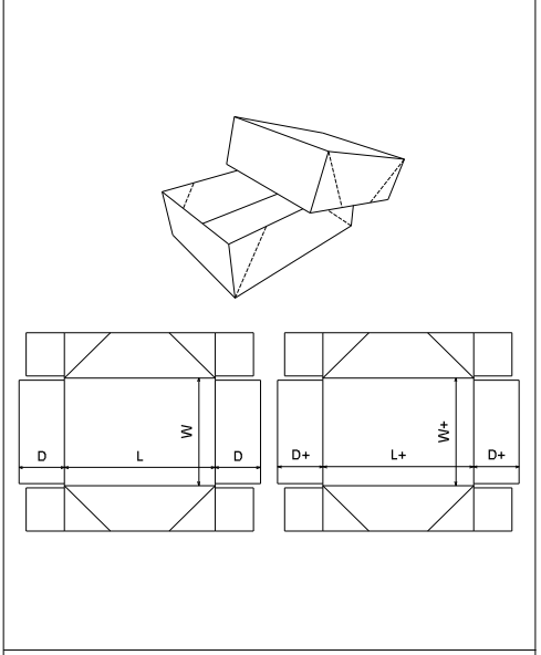
FEFCO 0303
