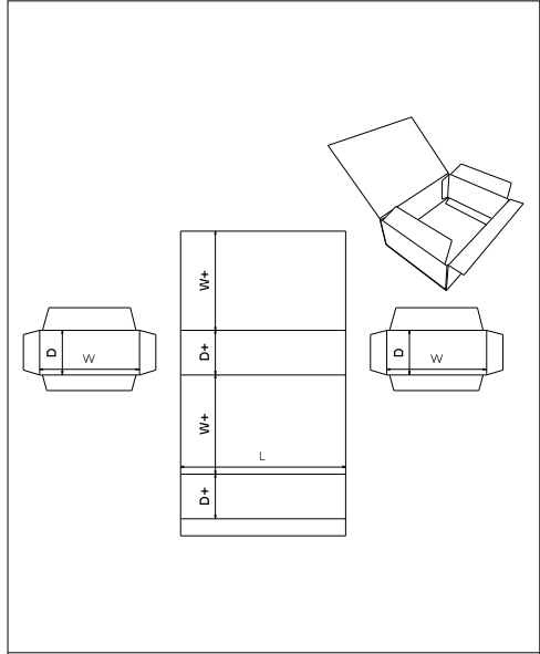
FEFCO 0607
