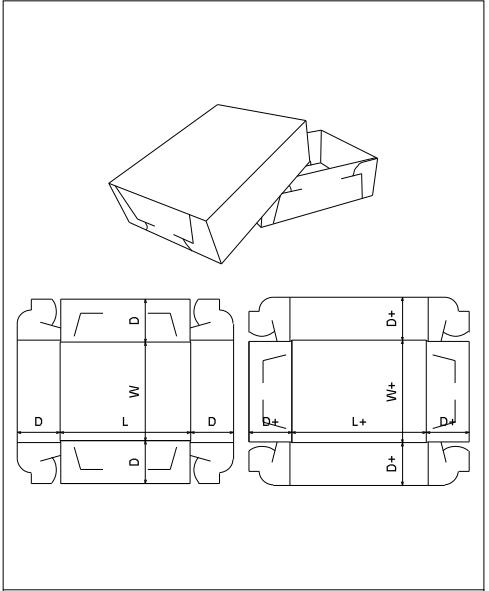
FEFCO 0307
