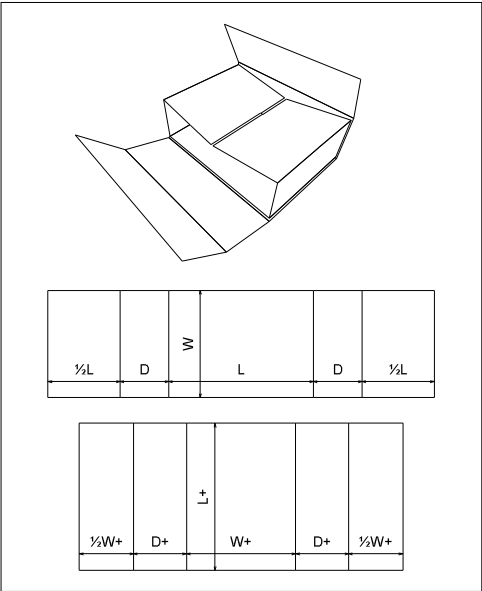
FEFCO 0404
