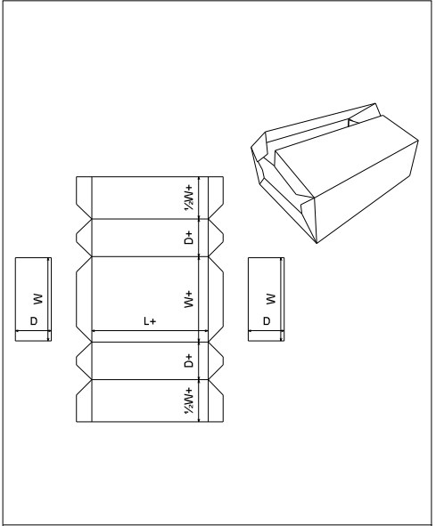
FEFCO 0606
