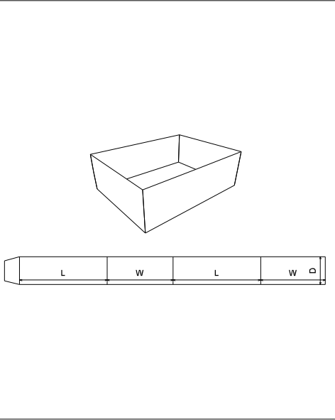
FEFCO 0501
