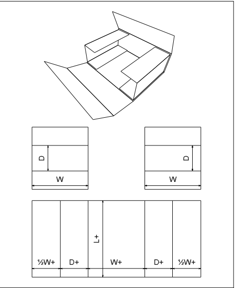
FEFCO 0405
