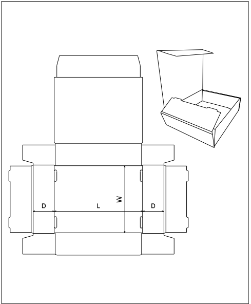
FEFCO 0421
