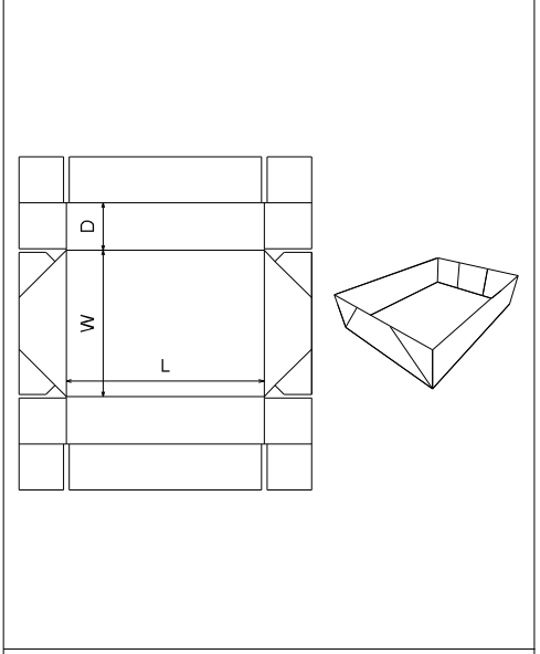
FEFCO 0718
