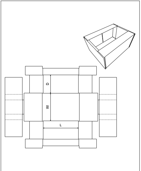
FEFCO 0433
