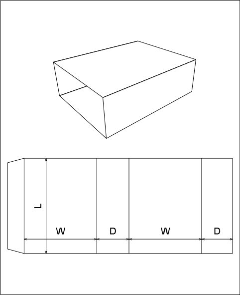
FEFCO 0503
