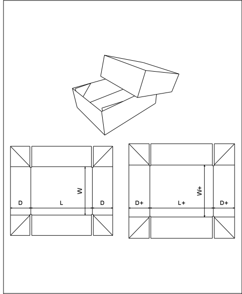
FEFCO 0308
