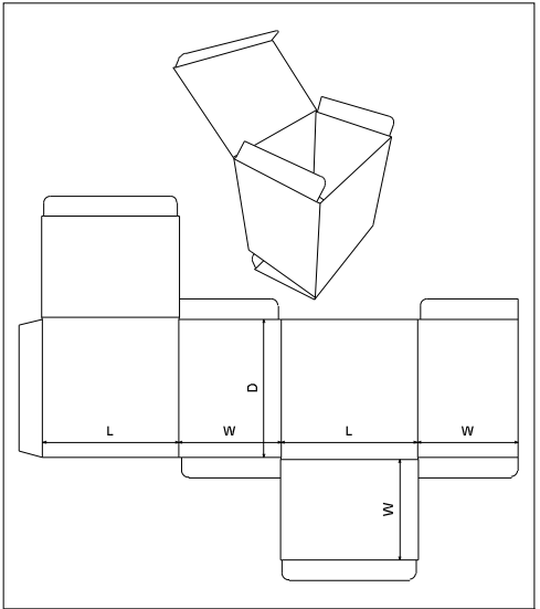
FEFCO 0211
