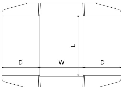
FEFCO 0460
