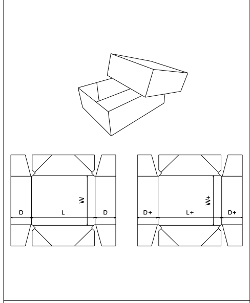
FEFCO 0304
