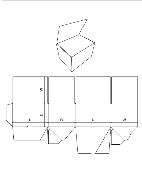
FEFCO 0703
