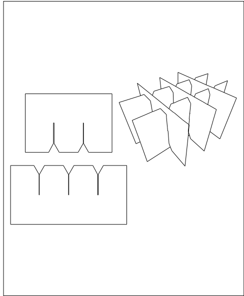
FEFCO 0933
