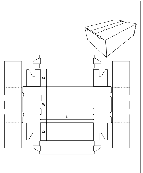
FEFCO 0432
