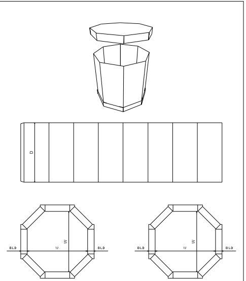
FEFCO 0350
