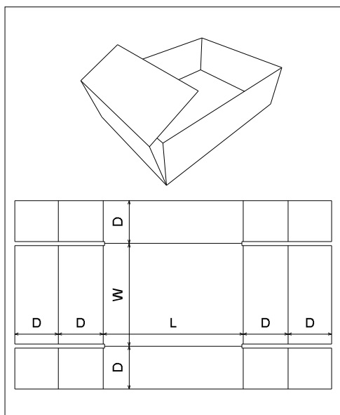
FEFCO 0454
