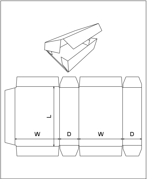
FEFCO 0406
