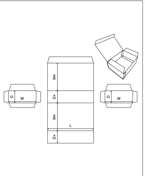
FEFCO 0608
